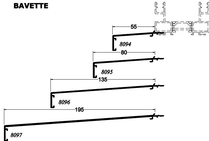
SEUIL PMR
