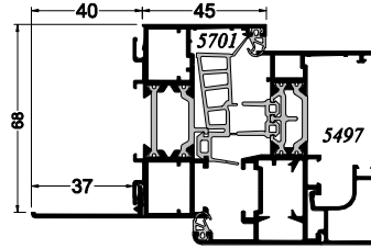
Ouvrant Visible (joint thermique)
