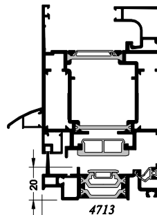
PE 4700 (plane)
