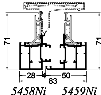
Traverse fixe dormant caché
