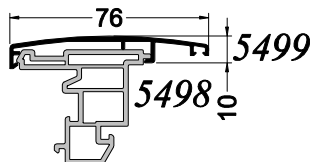
Ouvrants visibles Classic
