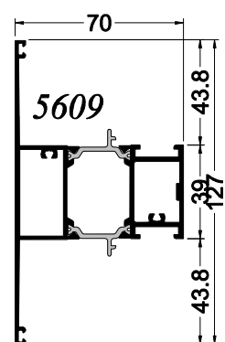
Meneau dormant caché
