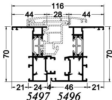
Traverses ouvrants visibles & dormants
