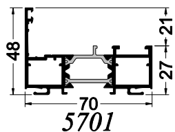
Ouvrants visibles Classic
