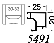
Parcloses dormants et ouvrants visibles
