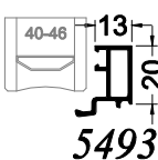
Parcloses dormants et ouvrants visibles
