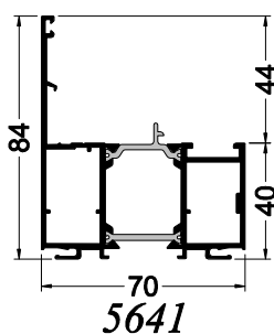
Ouvrants cachés
