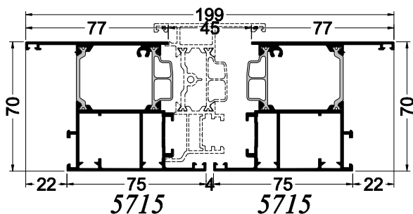
Parcloses dormants et ouvrants visibles
