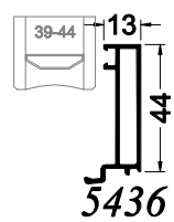
Parcloses dormant caché
