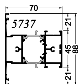
Traverse fixe dormant caché
