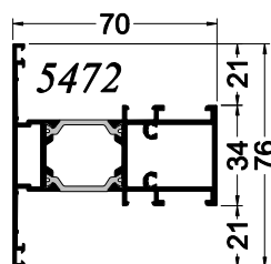
Traverses ouvrants visibles & dormants
