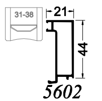
Parcloses dormant caché
